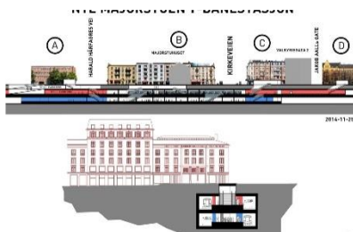
Ny to-etasjes stasjon Majorstuen
