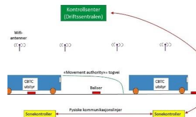
CBTC prosjektet Foregår parallelt i Sporveien. Fornebu-banen bekoster sin del.
